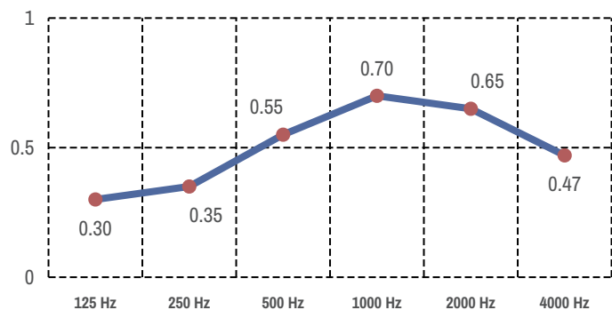
Gráfico de Absorción acústica
