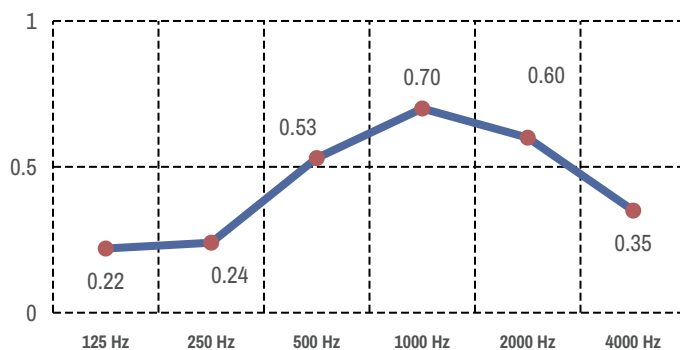
Gráfico de Absorción acústica (NCR e = 16mm)
